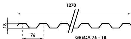
Greca 76-18
